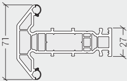
LCW9021 Zero|90 Transom T
