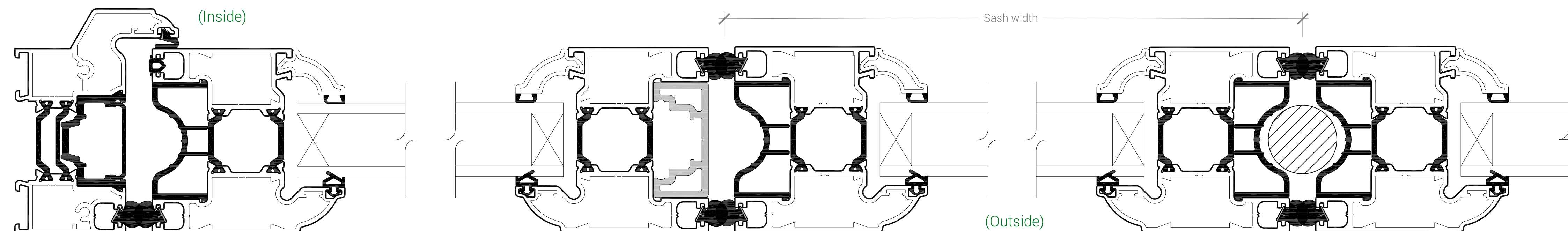
SECTION 'B-B'
