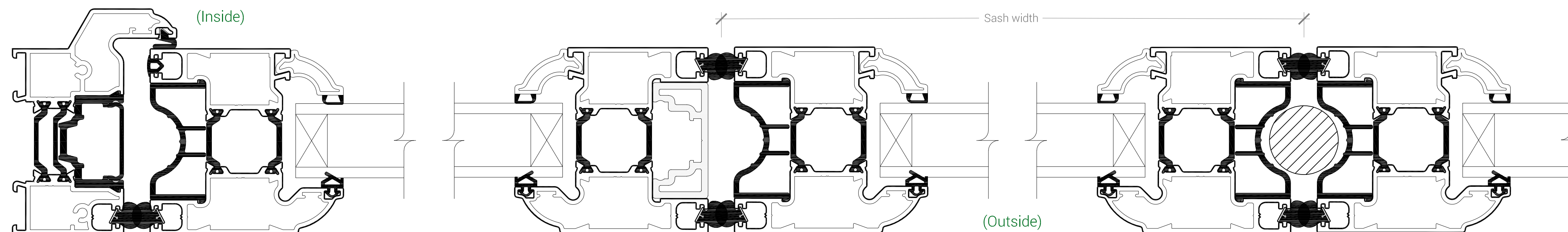
SECTION 'B-B'
