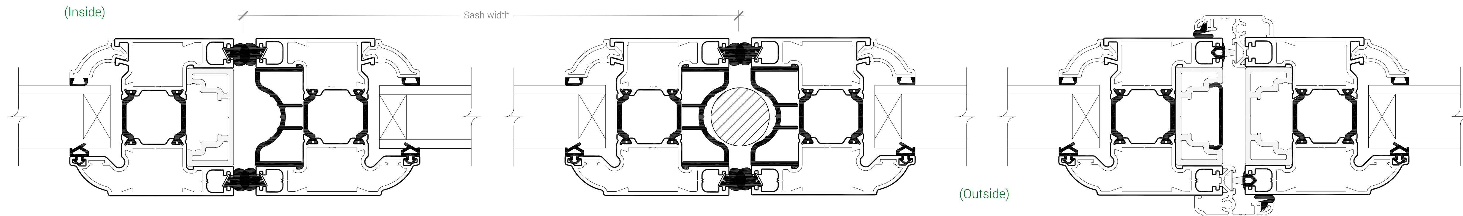
SECTION 'B-B'
