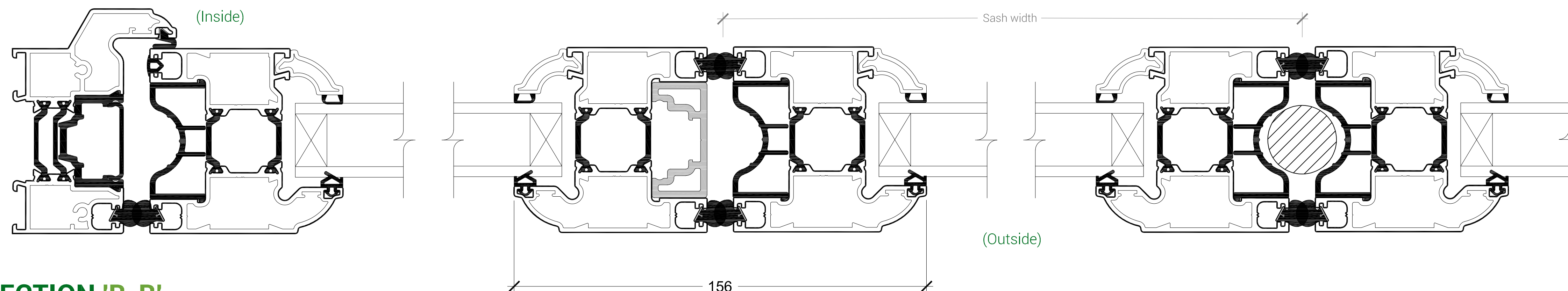
SECTION 'B-B'
