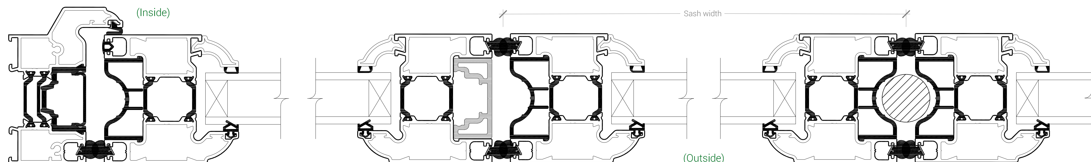
SECTION 'B-B'
