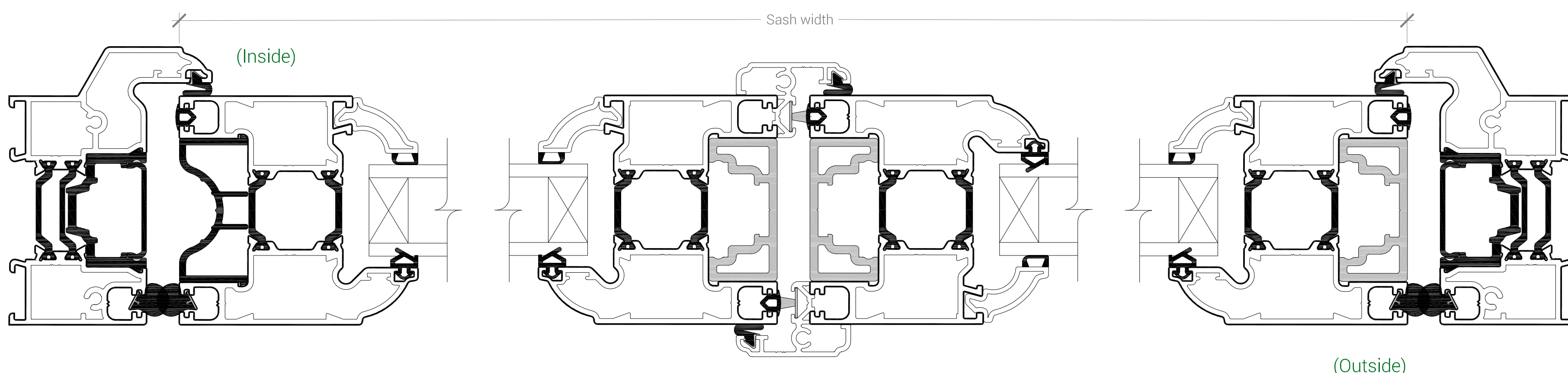
SECTION 'B-B'
