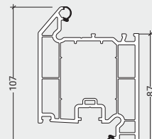
SLCW037 Door Sash Z
