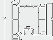
LSW036 Door Sash T
